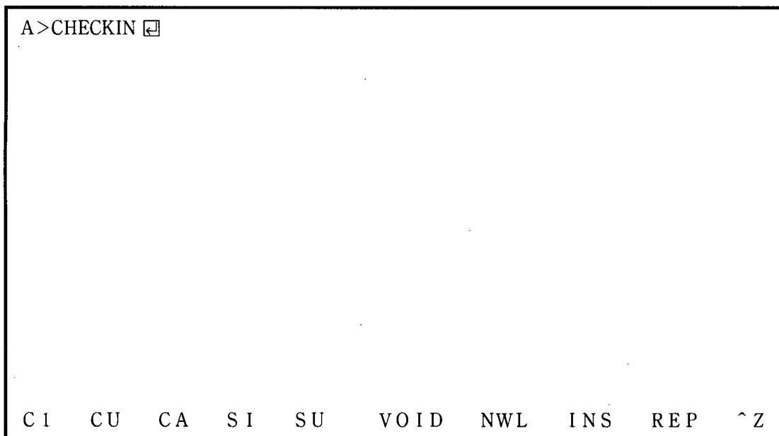
Fig. 19 利用者データの登録を行うためのプログラム名を入力し、起動している画面 “A>” に対し、CHECKIN と入力する。 “CHECKIN.EXE” は利用者登録を行うためのプログラム名である。
